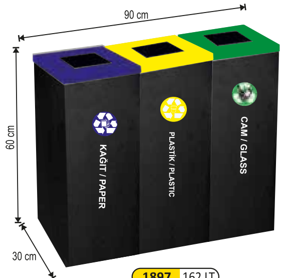
1897 162 LT 3LÜ BOYALI GERİ DÖNÜŞÜM KOVASI 54 LT PAINTED RECYCLING SET WITH LID 3 BUCKETS 3-х ведерная сортировочная урна, крашенная с крышкой, 54 л.
