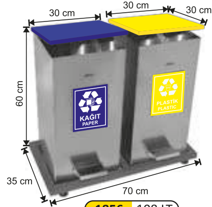
1856 108 LT. İKİLİ GERİ DÖNÜŞÜM ÇÖP KOVASI 2 BUCKET 108 LT STAINLESS STEEL RECYCLING PEDAL BIN 2-х ведерная сортировочная нержавеющая урна с педалью 108 л
