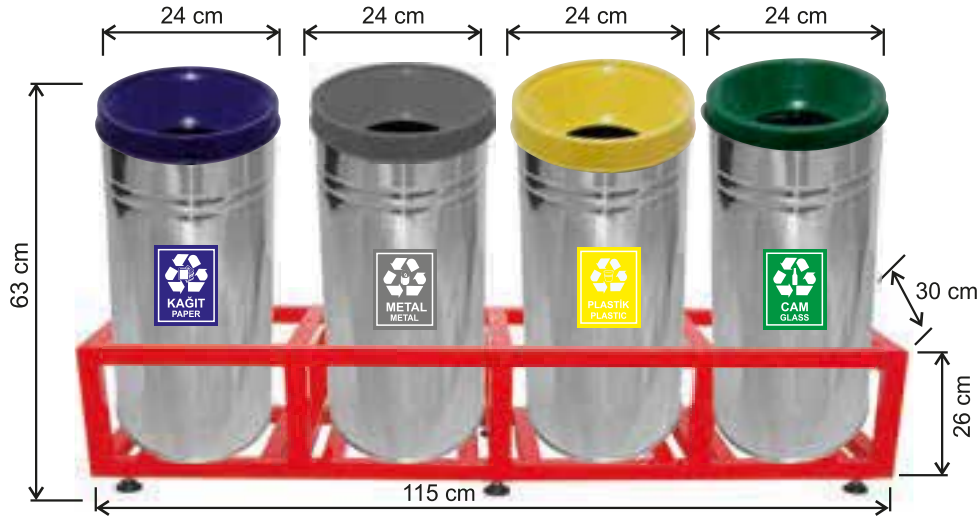
1812 GERİ DÖNÜŞÜM GRUBU 430 KALİTE (KAFESLİ) STAINLESS STEEL 4 BUCKET RECYCLING WASTE BIN WITH CAGE Сортировочная нержавеющая урна в защитной клетке с четырьмя ведрами
