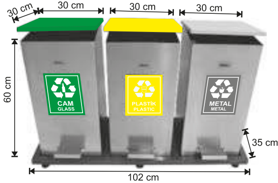
1857 GERİ DÖNÜŞÜM GRUBU 430 KALİTE MAT PASLANMAZ PEDALLI 3 BUCKET 108 LT STAINLESS STEEL RECYCLING PEDAL BIN 3-х ведерная сортировочная нержавеющая урна с педалью
