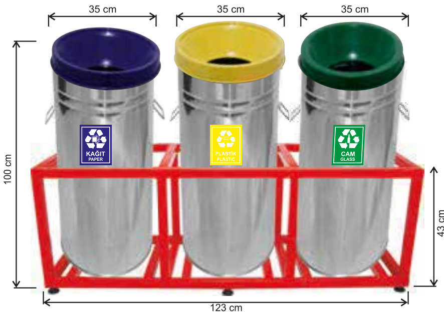
1811 GERİ DÖNÜŞÜM GRUBU PASLANMAZ (KAFESLİ) STAINLESS STEEL RECYCLING GROUP WITH CAGE 100X123 Сортировочная нержавеющая группа в защитной клетке
