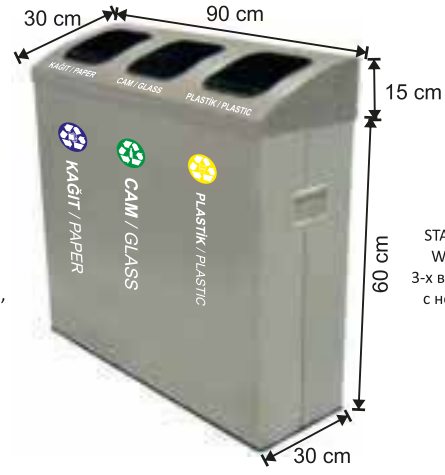
1807 235 LT. ÜÇLÜ GERİ DÖNÜŞÜM ÇÖP KOVASI STAINLESS STEEL RECYCLING SET WITH LID 3 BUCKETS 3-х ведерная сортировочная урна, с нержавеющей крышками
