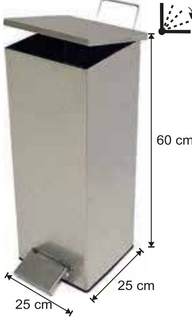
1082 34 LT AMORTİSÖRLÜ KARE PEDALLI ÇÖP KOVASI 34 LT INDUSTRIAL TYPE SQUARE SHAPE PEDAL BIN Урна с педалью индустриального типа 34 л
